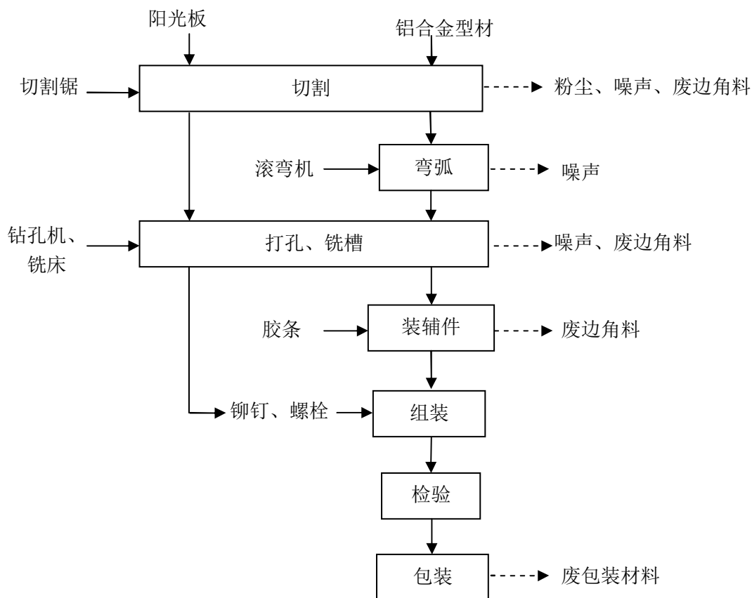
图 5-3 雨棚生产工艺流程及产污节点图
