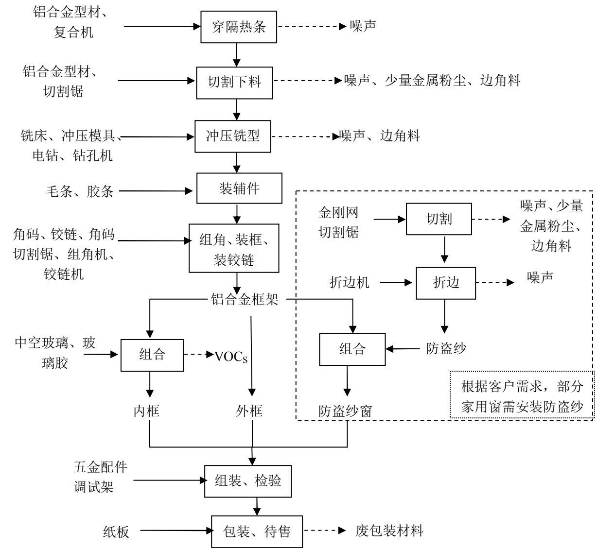
图 5-2 铝合金门窗加工工艺流程及产污节点图
