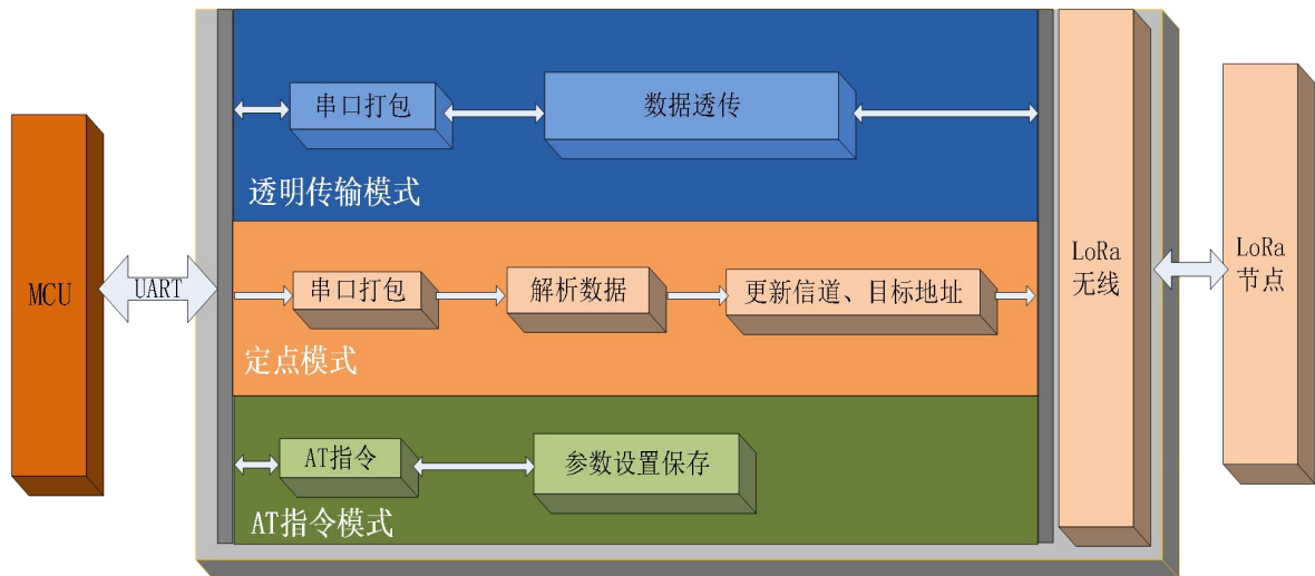
图 1 功能框图
