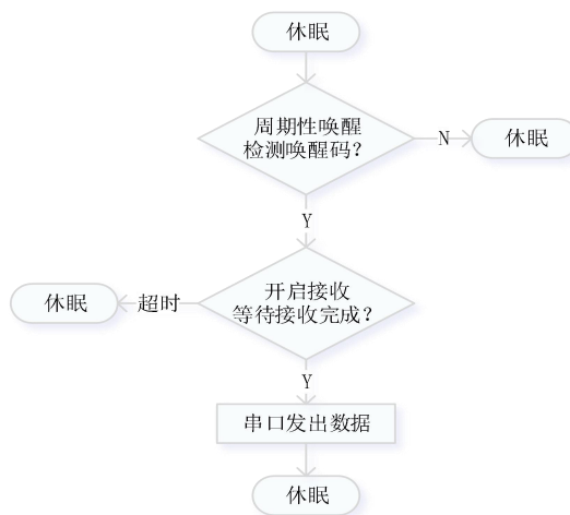
图 5 LR 模式工作流程
