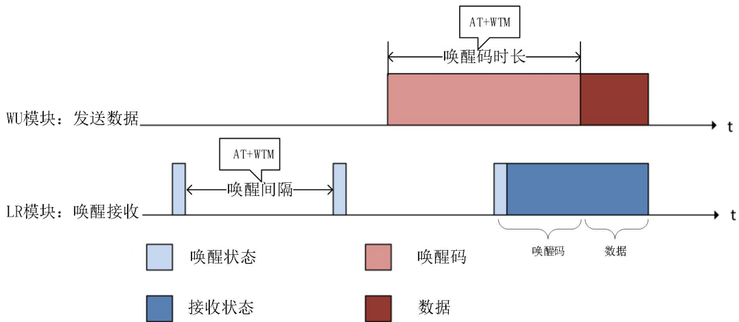
图 4 WU 和 LR 模式工作流程
