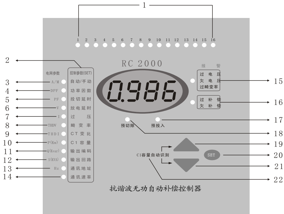
开孔尺寸为140mm×140mm型面板功能图
