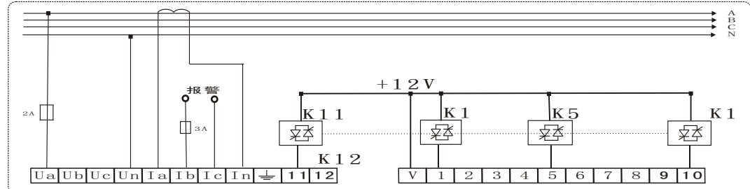
RC2000S动态接线图
