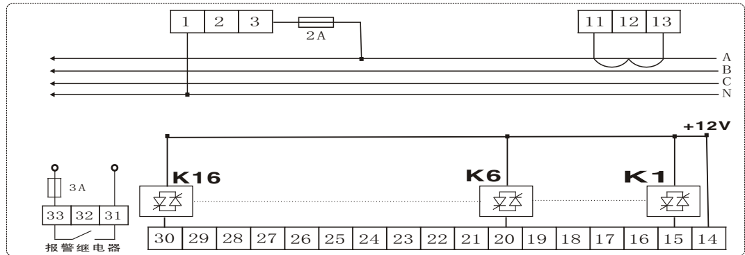
RC2000动态接线图
