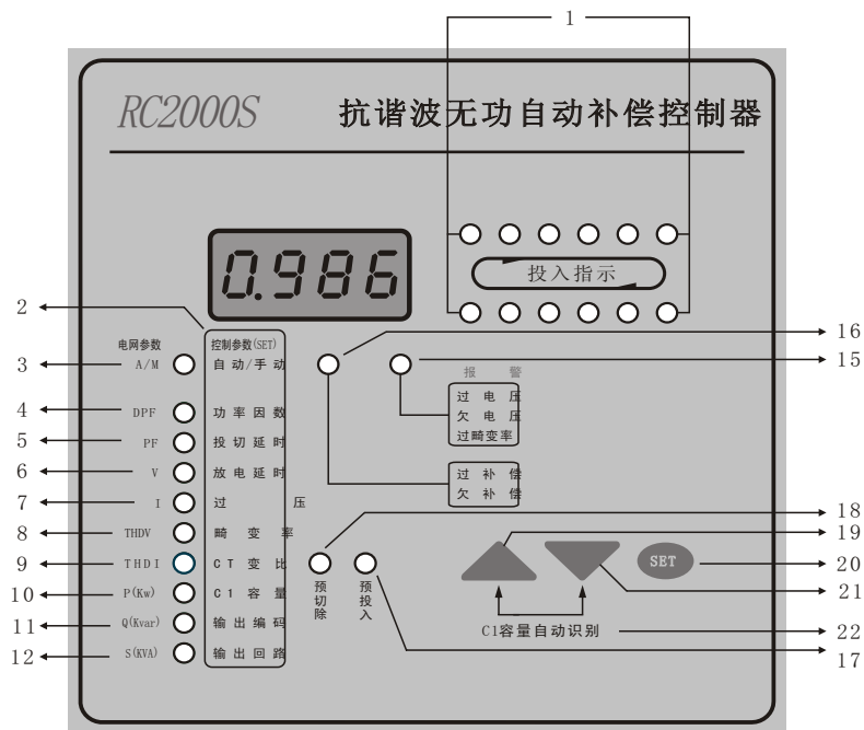
开孔尺寸为113mm×113mm型面板功能图
