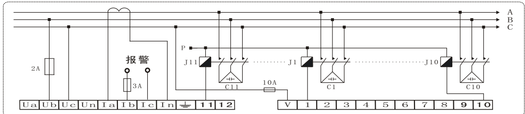
RC2000X-PP-XXS型开孔尺寸为113mm×113mm接线图
