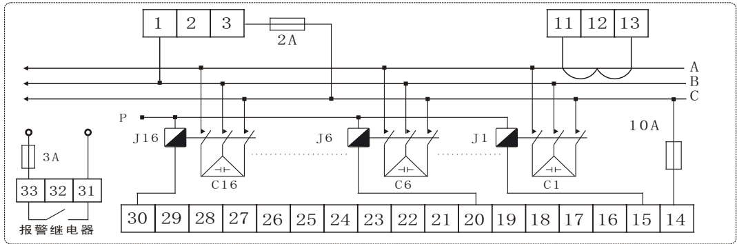
RC2000X-PP-XX型开孔尺寸为140mm×140mm接线图
