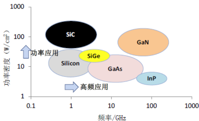
图 19：化合物半导体应用
