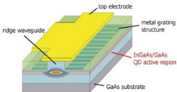
图 20：反馈激光器
