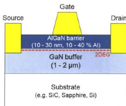
图 32：AlGaIn/GaN HEMT 截面图
