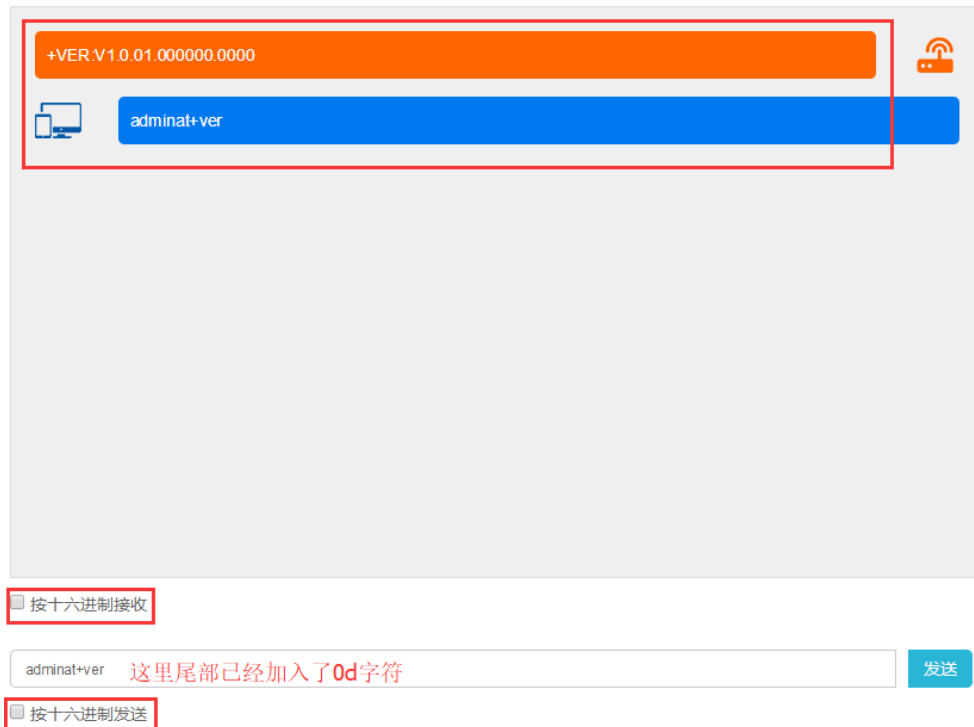
图 13 命令交互
