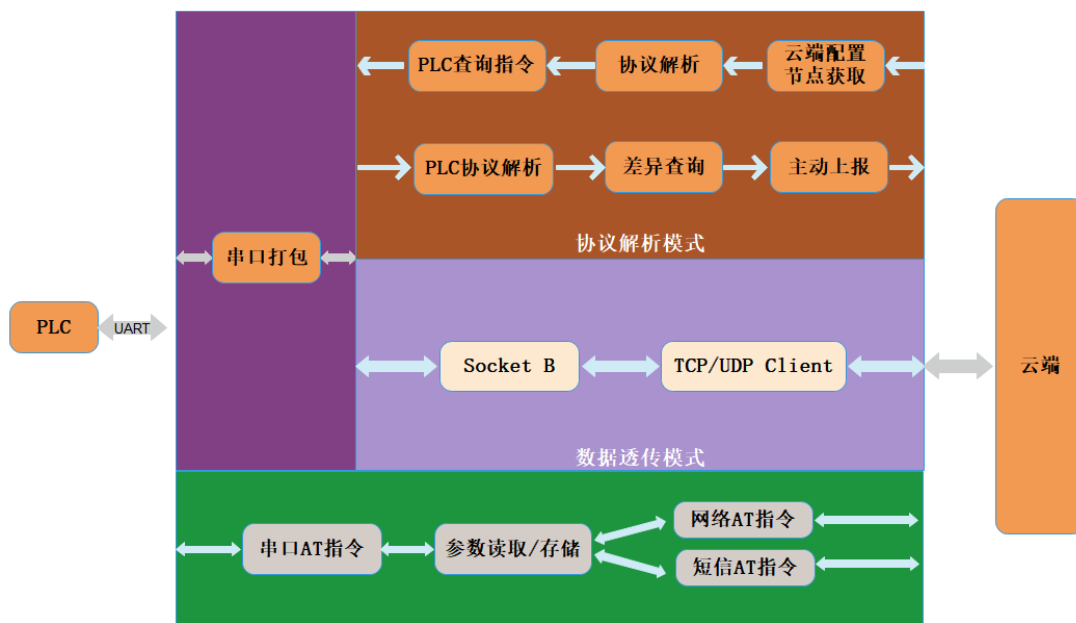
图 2 功能框图
