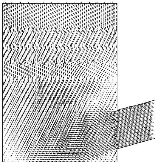
图 2 气相湍流速度场
