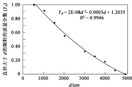
图1 喷淋液滴粒径 Rosin-Rammler 分布
