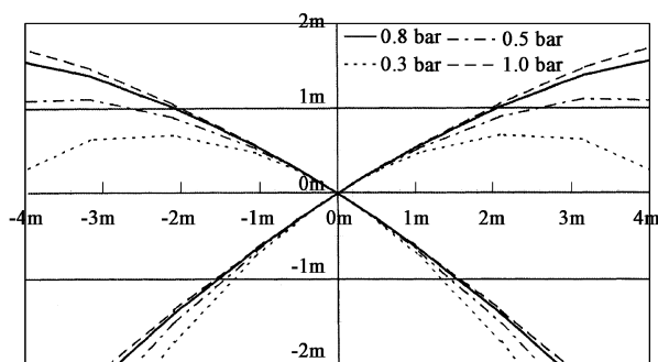
图6 喷淋范围实验曲线
