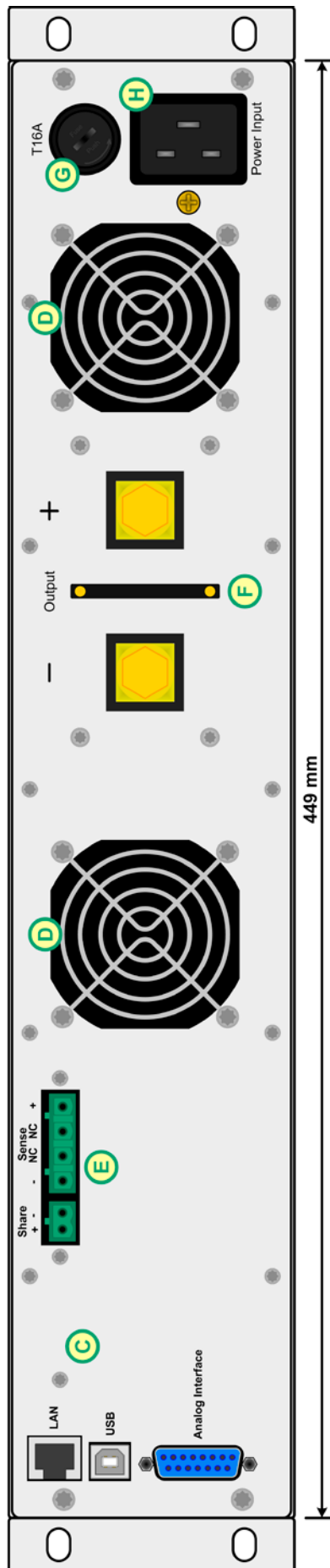
图 2 - 后视图
