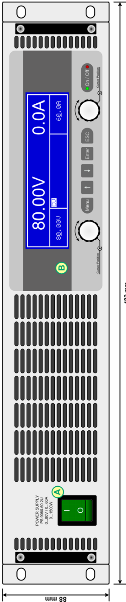
图 1 - 前视图
