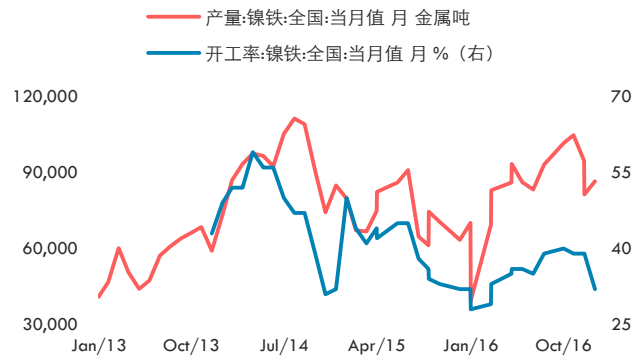
图 18: 镍铁产量 单位: 吨/月
