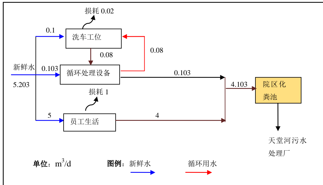
图 1 建设项目水量平衡图
