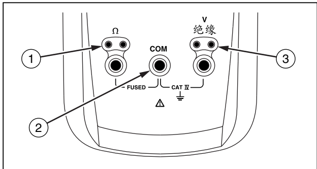
图 4. 输入端子
