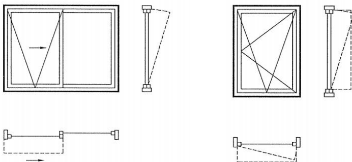
图 10 推拉下悬窗开启方式示意图 图 11 平开下悬窗开启方式示意图
