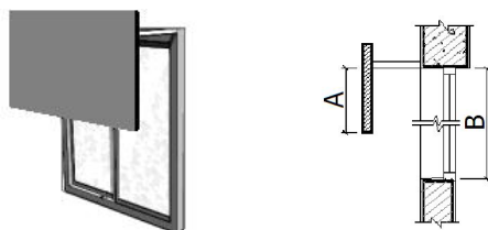
图 E.0.1-3 挡板式遮阳
