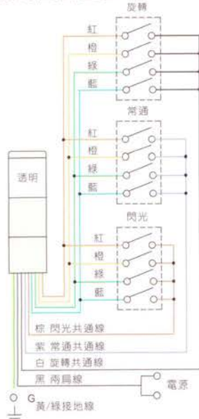
旋轉閃光型 (RF)
