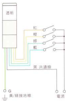
閃光蜂鳴型 (MS)
