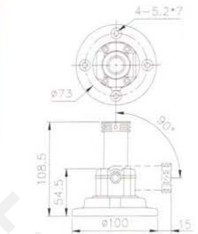
TPTL6-F (新型式專利, 圓形塑膠盤) 使用於TPFS4/TPFF4/TPFB4 TPF□5/TPF□6/TPF□7
