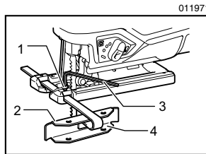
1. 螺栓 2. 切锯导板导向板 3. 六角扳手 4. 切锯导板（导尺）
