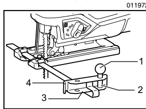
1. 螺纹旋钮 2. 销 3. 切锯导板（导尺） 4. 切锯导板导向板
