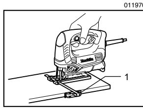
1. 切锯导板（导尺）
