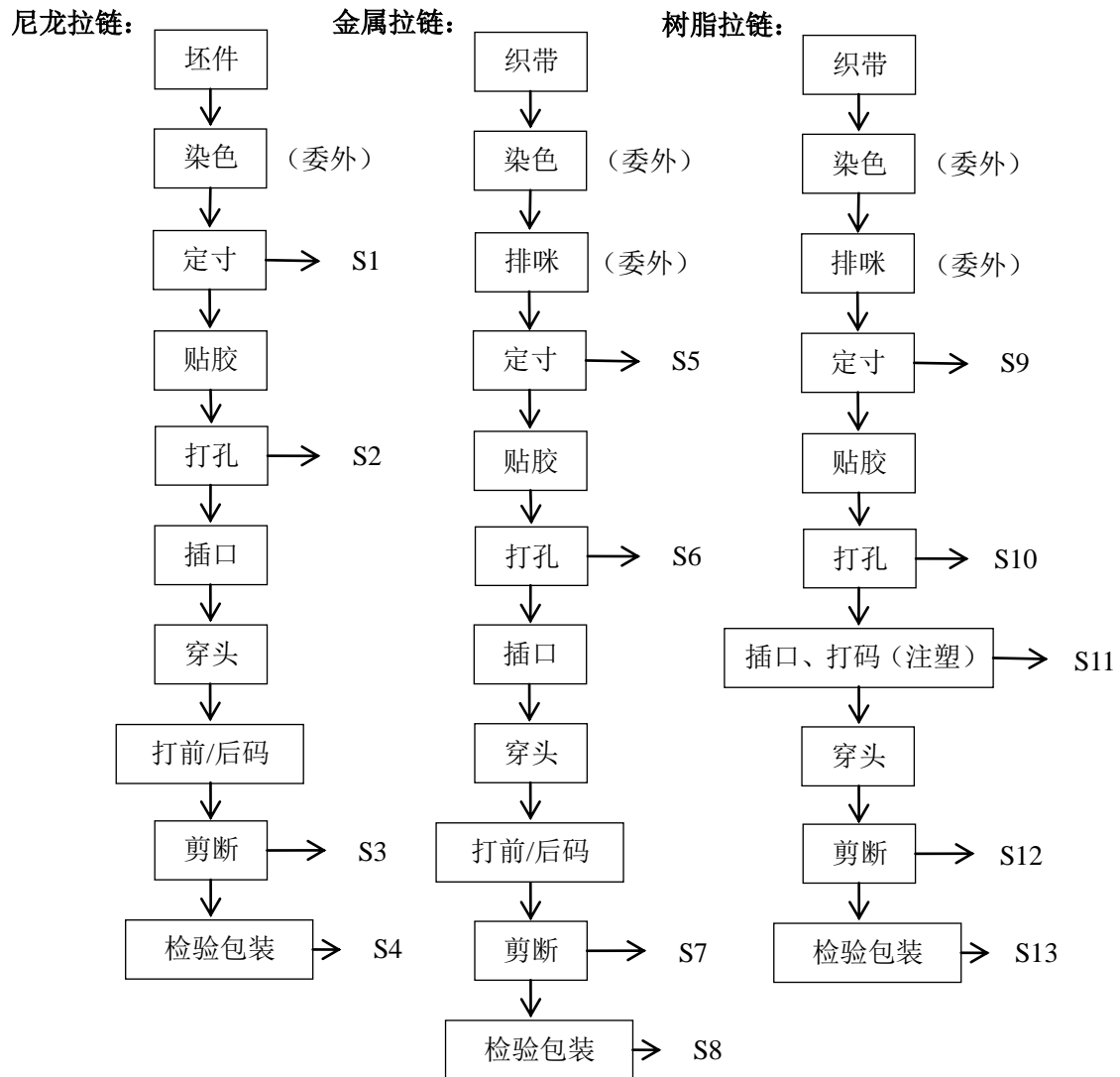
图 5-1 生产工艺流程图
