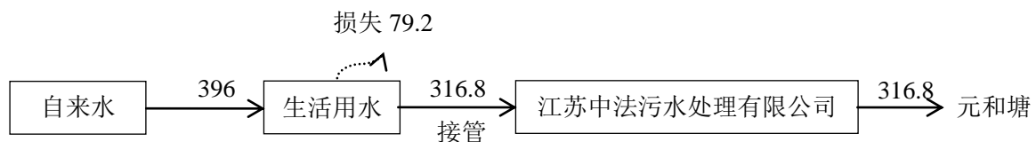
图 5-2 水量平衡图
