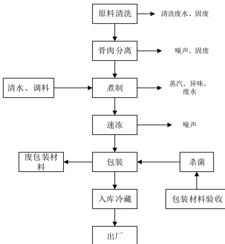
图 5-2 营运期工艺流程及产污环节分析图
