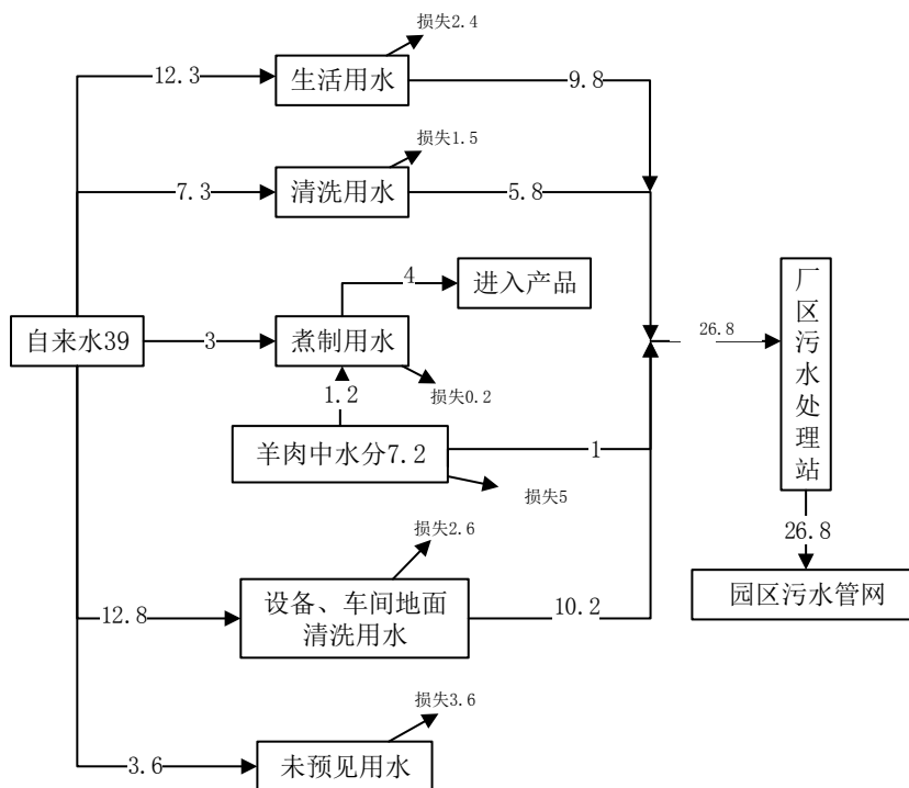
图 5-5 本项目水平衡图
