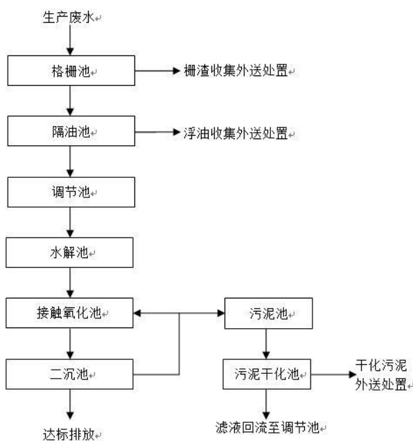
图 5-6 本项目污水处理工艺流程图
