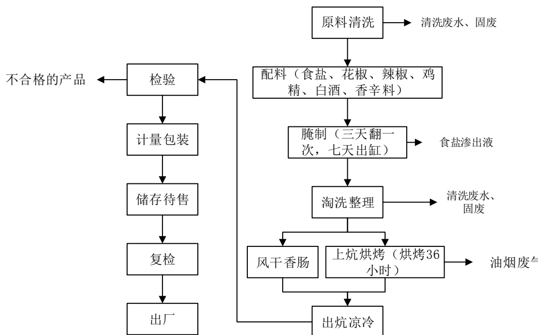
图 5-3 营运期羊肉风干香肠工艺流程及产污工序图
