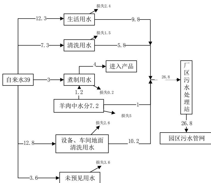
图 5-4 本项目水平衡图
