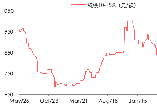
图 3: 镍铁价格
