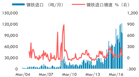
图 4: 镍铁进口量
