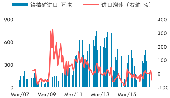
图 2: 镍矿进口
