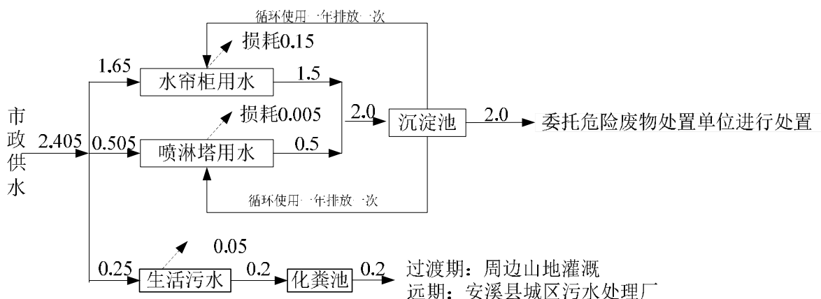
图 5-1 项目扩建工程水平衡图 单位：t/d
