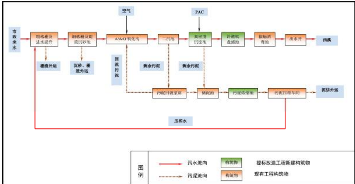
图 3-1 安溪县城市污水处理厂工艺流程图
