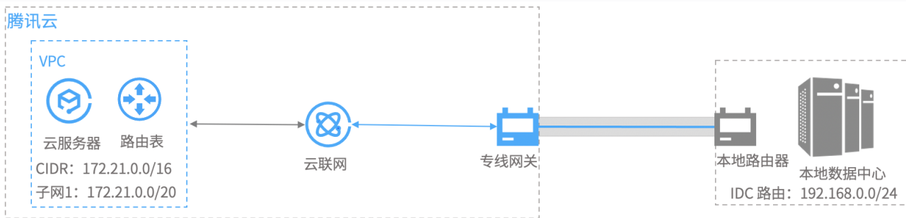
VPC 路由表
