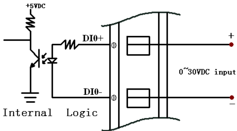
外部接线图（外接 0~30V 电压）
