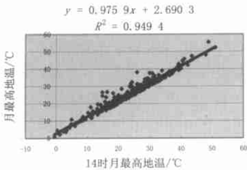
图 3 月最高地温与 14 时月最高地温之间的关系
