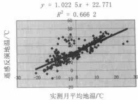
图 1 遥感反演地温与实测月平均地温的关系
