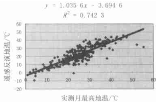
图 2 遥感反演地温与实测月最高地温的关系
