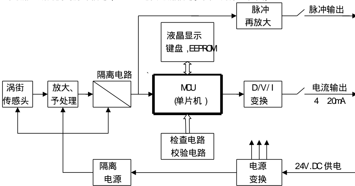
图 1 涡街流量计原理框图
