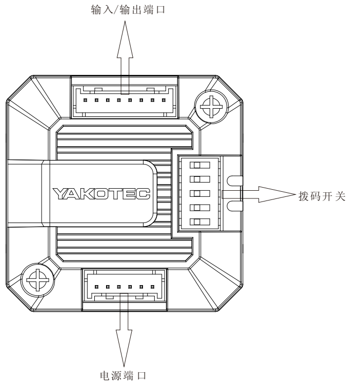
接线示意图
