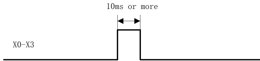
X0-X3 时序图
