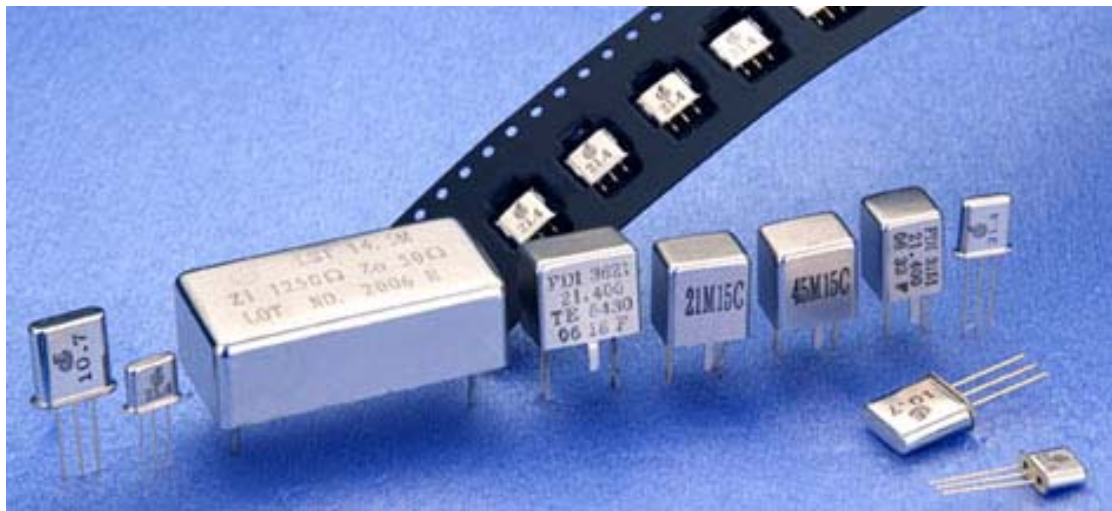
晶体滤波器
