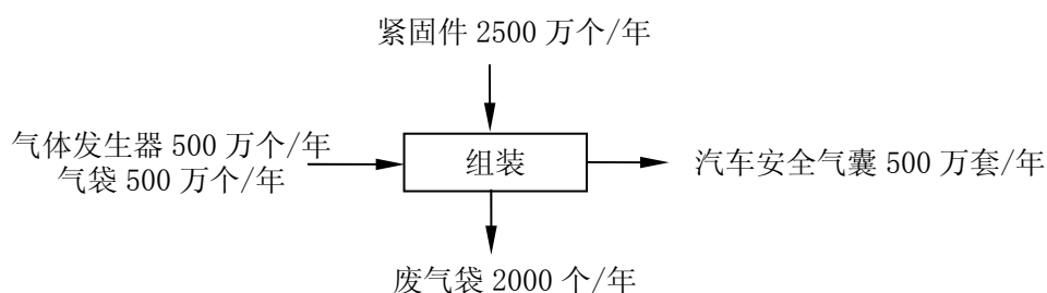
图 1 本项目产品生产工艺流程图
