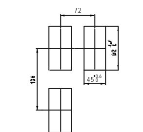
XMT-420D/S 开孔尺寸
