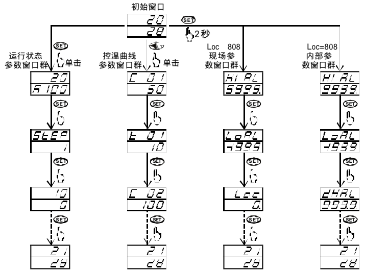
各参数窗口群间的转换示意图
