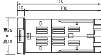
XMT-420C 外形尺寸
