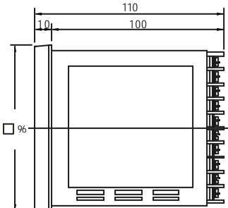
XMT-420D/S 外形尺寸
