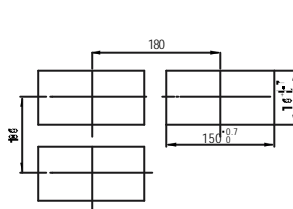
XMT-420A 开孔尺寸
