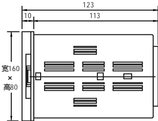
XMT-420B 外形尺寸
