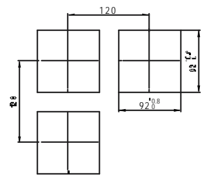
XMT-420B 开孔尺寸
