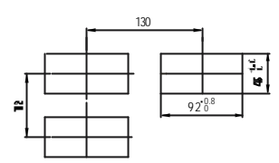
XMT-420C 开孔尺寸
