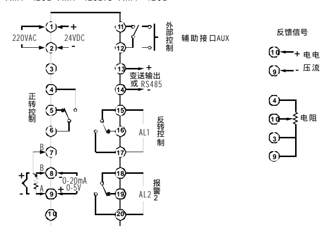
XMT-420B XMT-420D/S XMT-420D
