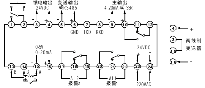
XMT-420B XMT-420D/S XMT-420D
