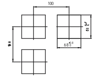
XMT-420C 开孔尺寸
