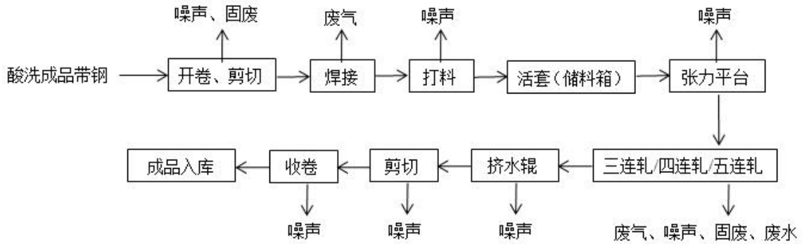
图 2-3 冷轧生产工艺流程及产污节点图
