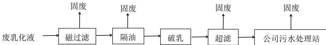
图 2-4 供水站工艺流程产污环节示意图
