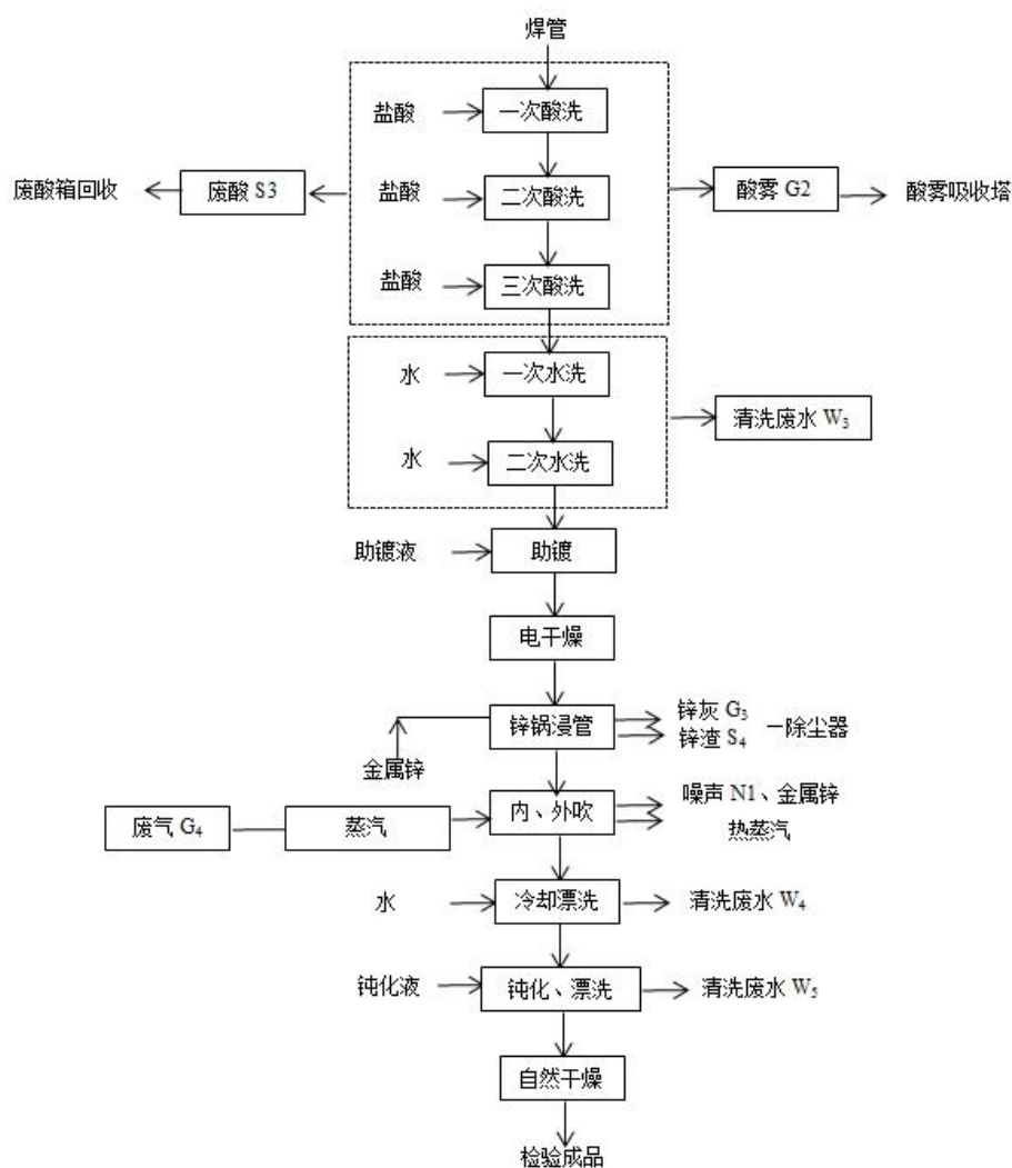
图 2-2 镀锌工艺流程产污环节示意图
