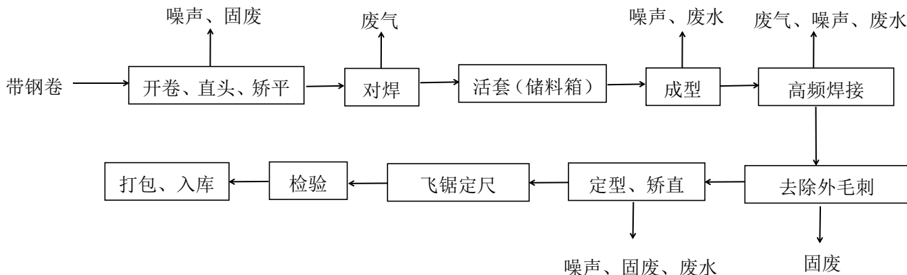
图 2-1 焊管生产工艺流程及产污节点图
