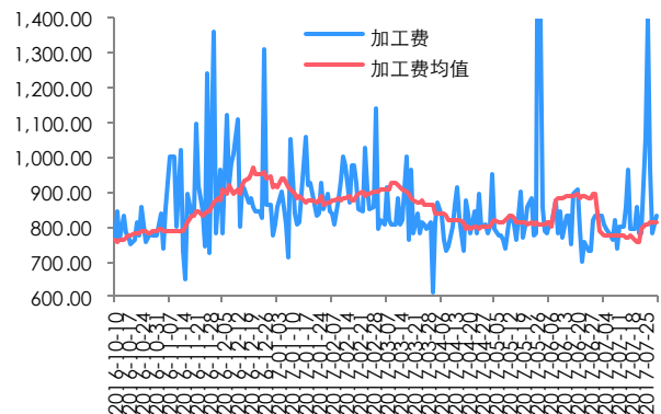
图 4：铜杆加工费
