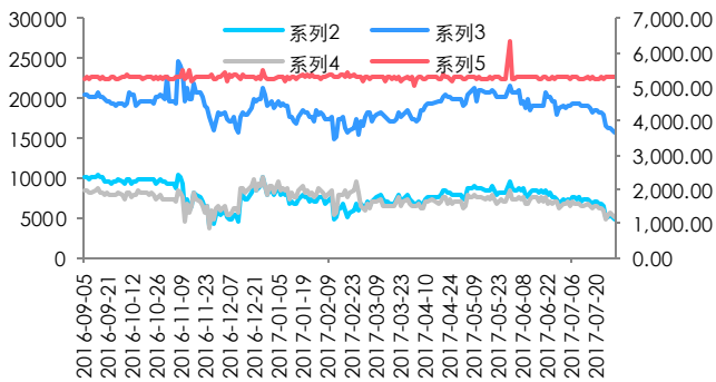
图 3：线缆利润
