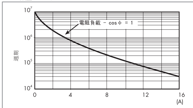
F 45 - 電氣壽命 (AC) 與觸點電流 類型 45.31/45.91
