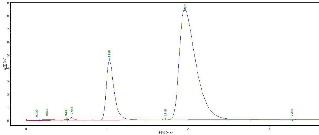
苯、甲苯分析色谱图:
