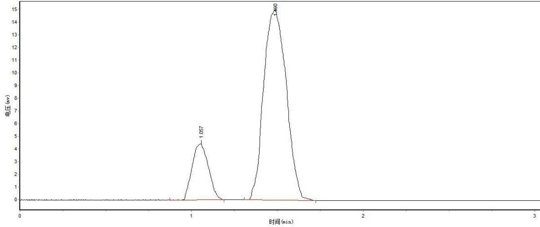
苯、甲苯分析色谱图:
