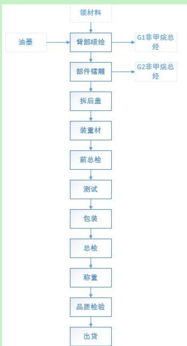
5-1 项目生产工艺流程图
