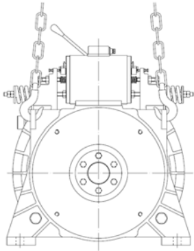
吊装示意图
