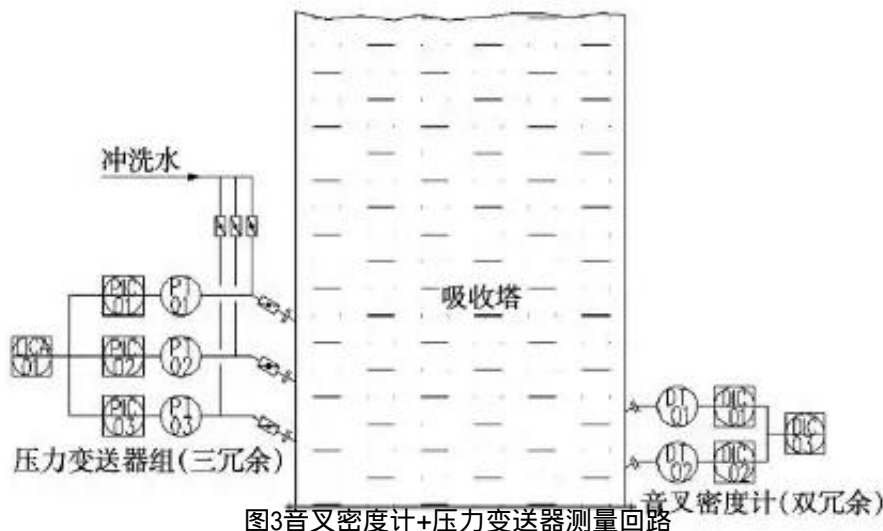
图3音叉密度计+压力变送器测量回路
