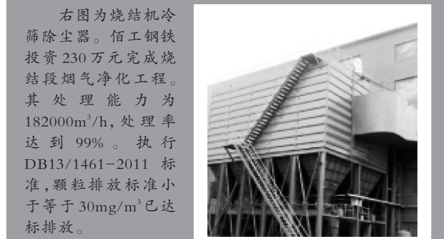
左图为烧结脱硫石灰-石膏湿法环保设施,其设计处理能力为960000m 3 /h;设计处理效率为95%;实际处理能力为960000m 3 /h;实际处理效率为95%;与主体设施的同步率为100%。
