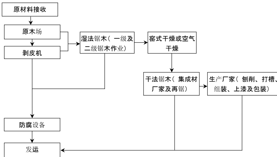
图 A.1 典型的锯木及木制品生产工艺
