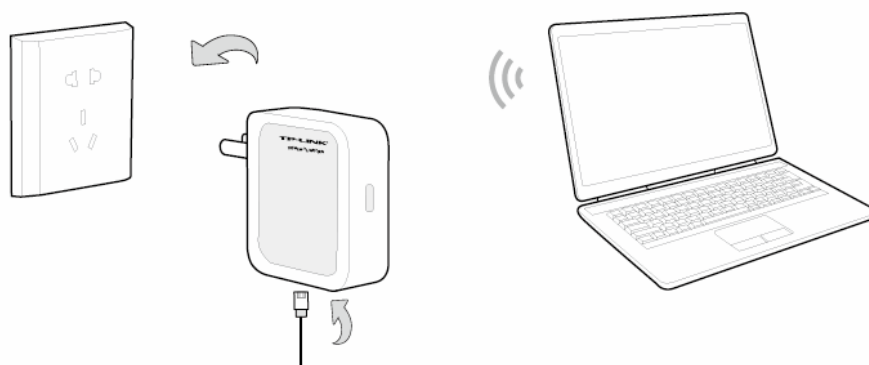
图 4-1 TL-WR700N 硬件安装示意图
