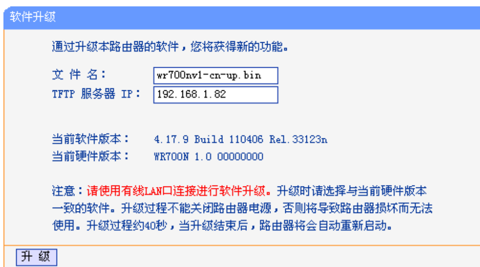
图 7-15 软件升级
