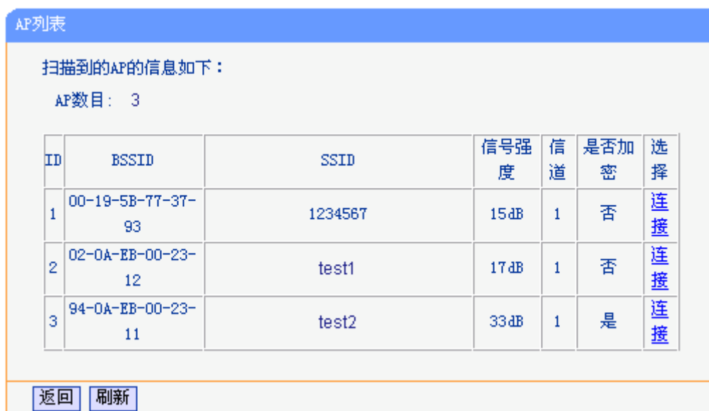
图 4-15 AP 列表
