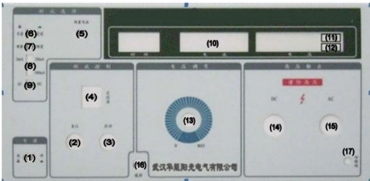
图(2) 数显式耐压测试仪前面板示意图
