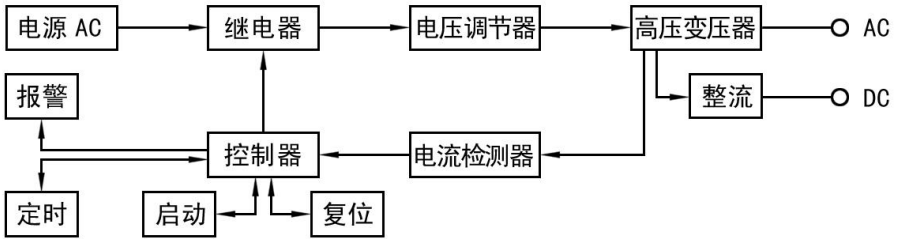
图(1):全数显耐压仪工作原理方框图
