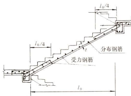
图 1 板式楼梯梯段
