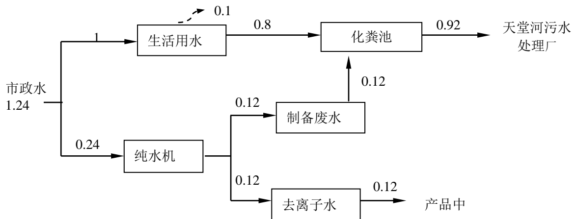
图 1 建设项目水平衡图 单位： \text{m}^3/\text{d} “ \dashrightarrow ”消耗量
