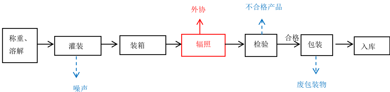
图 2-1 水凝胶产品（片状）工艺流程及产污节点图
