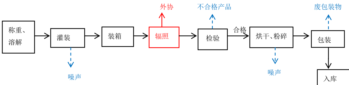
图 2-2 水凝胶产品（粉状）工艺流程及产污节点图
