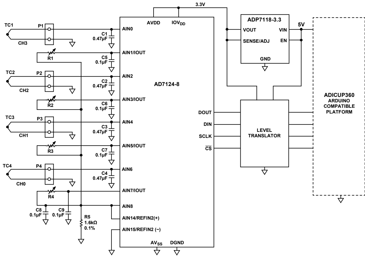
图1. 热电偶测量系统 (原理示意图: 未显示所有连接和去耦)
