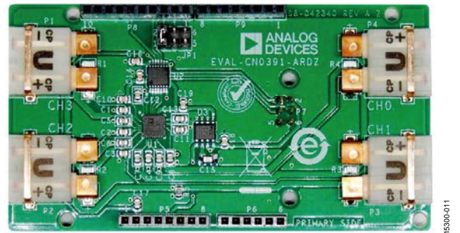
图 11 .EVAL-CN0391-ARDZ 板照片
