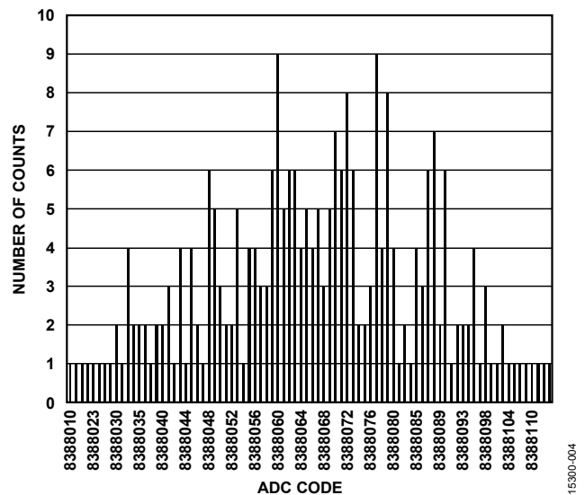
图4. 单通道的短路输入直方图，256 样本，ADC Sinc3 滤波器开启，50 Hz 数据速率
