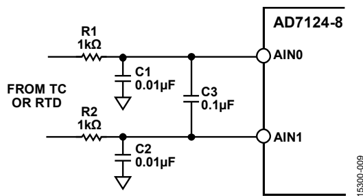
图 9. 适用于 AD7124-8 的可选差分与共模输入滤波器
