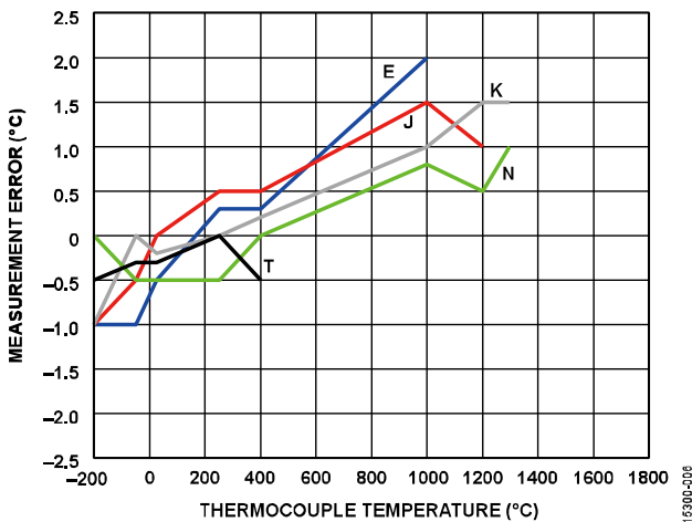
图6.EVAL-CN0391-ARDZ 温度测量误差 (E、J、K、N、T 型热电偶, 使用热电偶仿真器)
