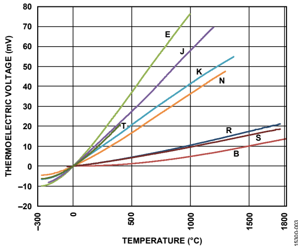
图3. 热电偶输出电压与温度的关系
