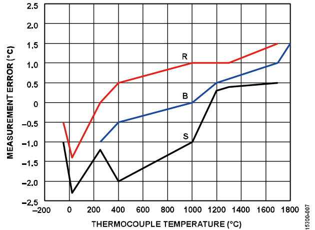
图7.EVAL-CN0391-ARDZ 温度测量误差 (B、R、S 型热电偶, 使用热电偶仿真器)
