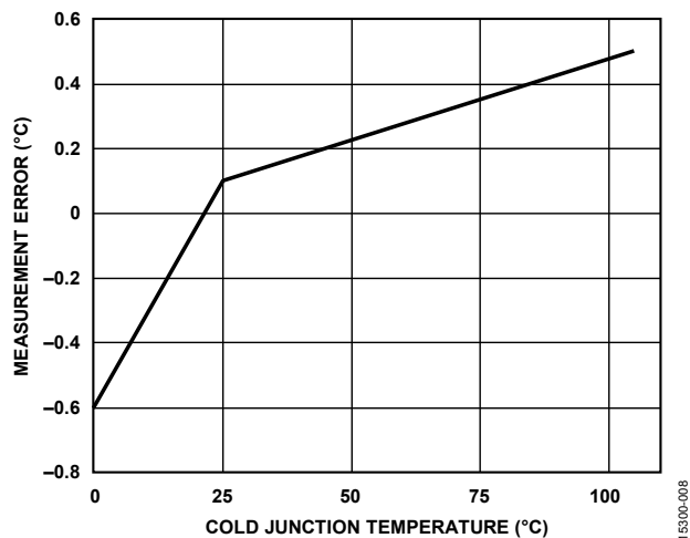
图 8. EVAL-CN0391-ARDZ 温度测量误差，J 型热电偶在室温下，冷端温度为 0°C、25°C 和 105°C
