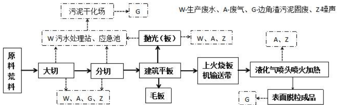
图 5-2 抛光、火烧板工艺流程及产排污节点图
