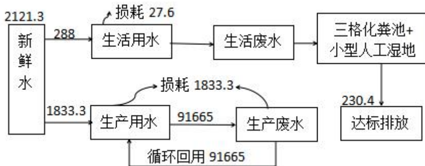
图 5-3 本项目水平衡图
