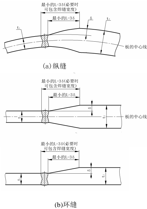
图 4-1 不同厚度钢板(元件的对接)
