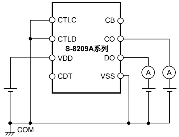
图14 测定电路8
