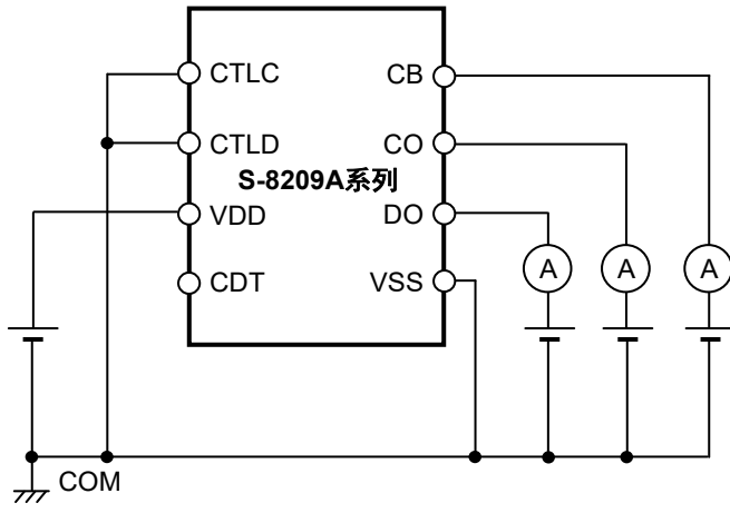
图13 测定电路7
