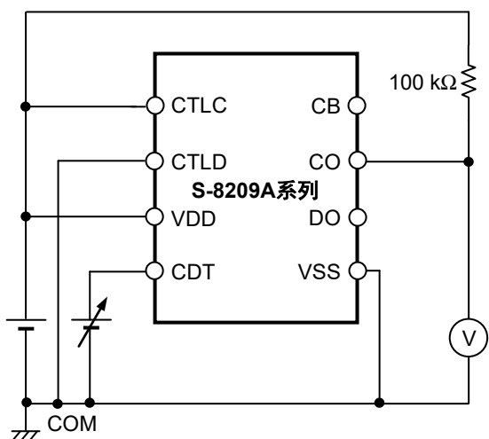
图9 测定电路3
