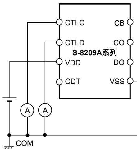
图12 测定电路6
