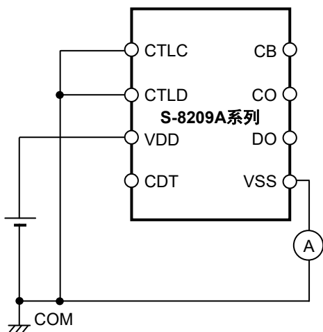
图11 测定电路5
