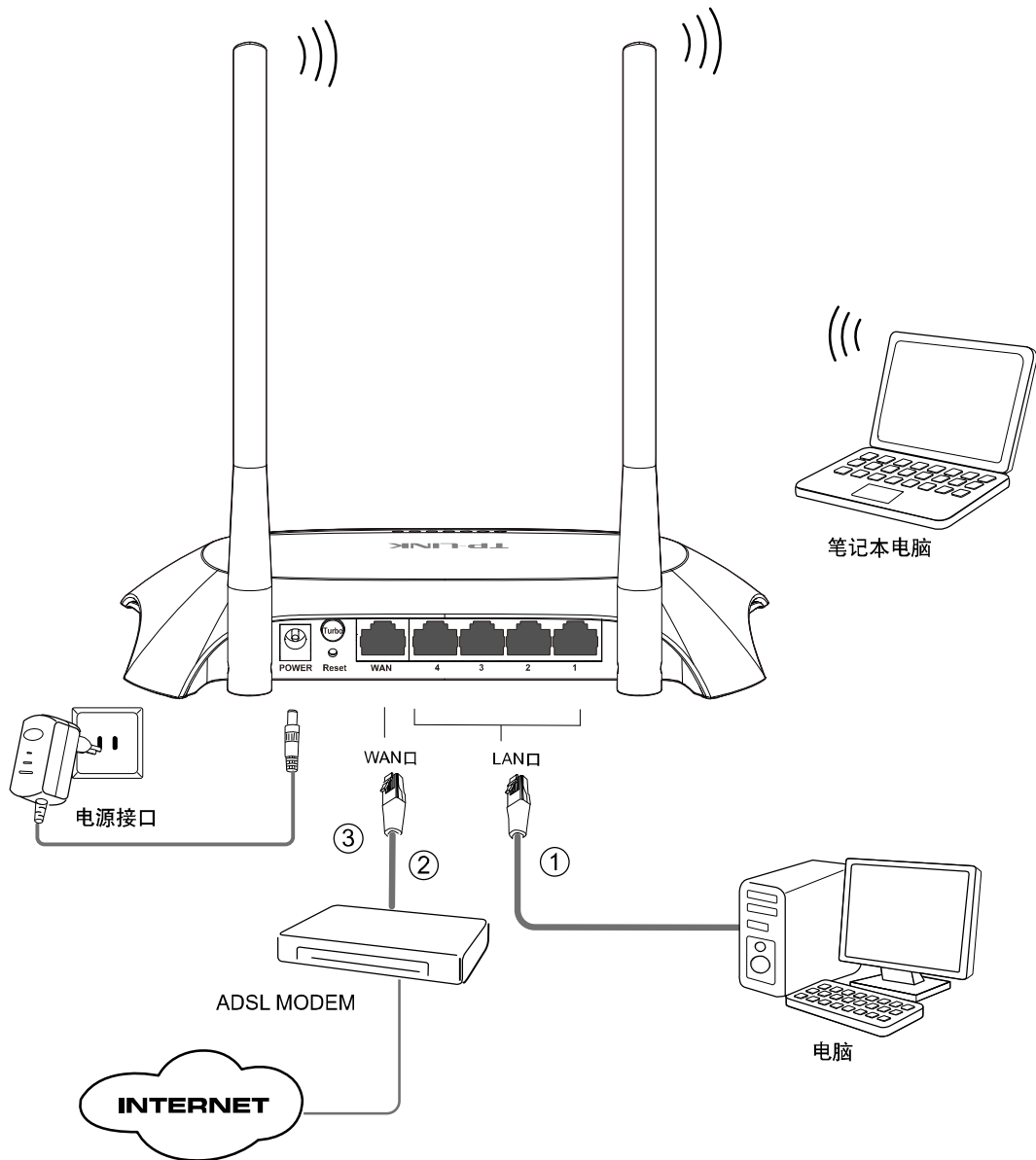
图4-1 TL-WR841N 硬件安装示意图
