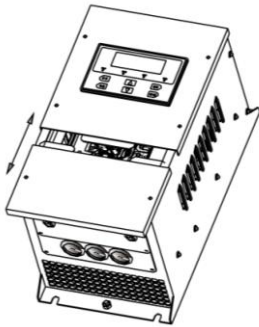
HFR2015-HFR2055 结构外观拆卸示意图
