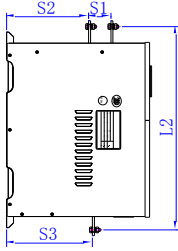
RC3 铜排结构尺寸
