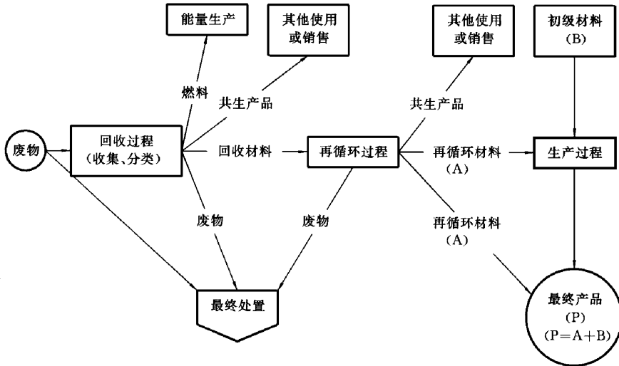
图 A1 再循环系统流程示意图
