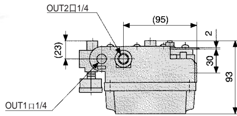
IP5000型(杠杆式杠杆反馈式)
