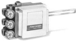
IP5000型(杠杆式杠杆反馈式)
