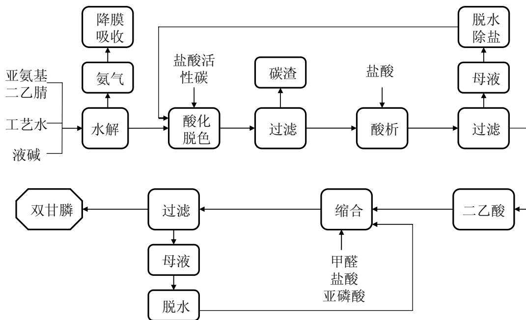
② 草甘膦生产流程图
