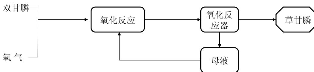
③ 吡啶生产流程图
