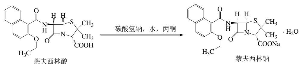
图 1-1 萘夫西林钠合成反应
