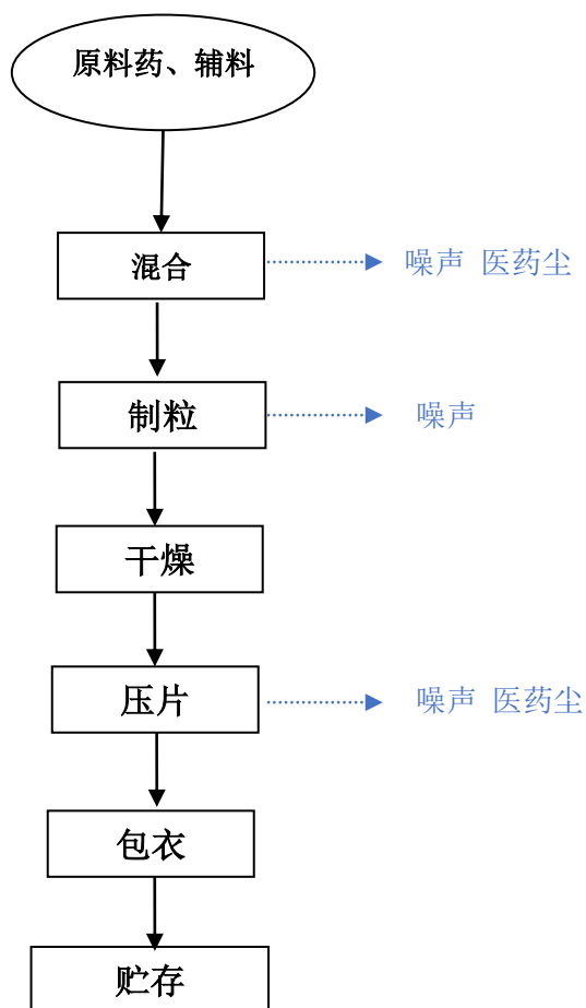
图 2-2 片剂制剂工艺及产污节点图
