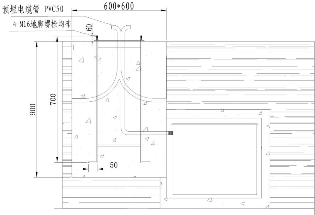
地脚螺栓详图
