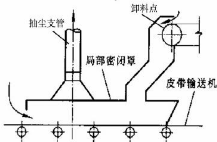
图 3-7 各皮带受料点除尘设施示意图
