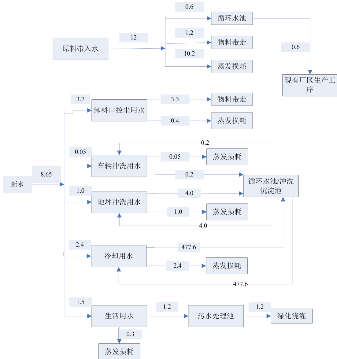
图3-5 项目水平衡图
